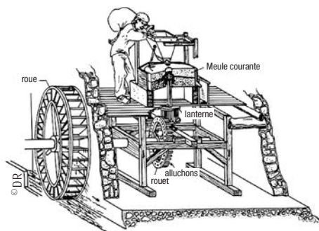
Fonctionnement d'un moulin à grain.
